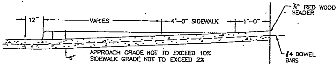
SECTION A-A
